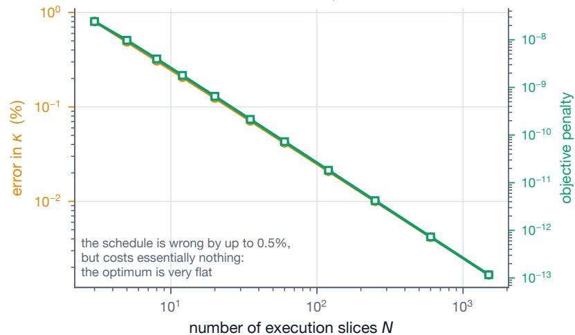
(d) Cost of the \kappa \approx \sqrt{\lambda \sigma^2 / \eta} approximation
