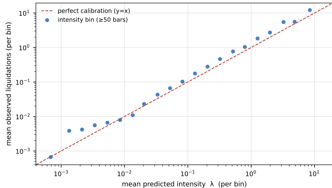
Aave v2 · branching n=0.63 (stationary ✓) · PIT KS D=0.0005
