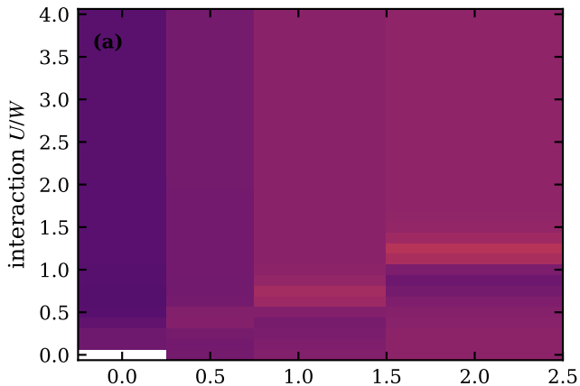
arith, n_c=0.26 , T/W=0.05 , \lambda=0
