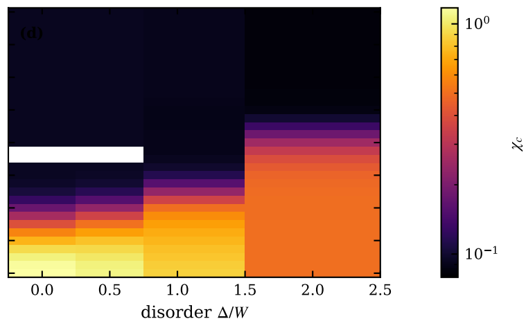
typ, n_c=0.49 , T/W=0.1 , \lambda=0
