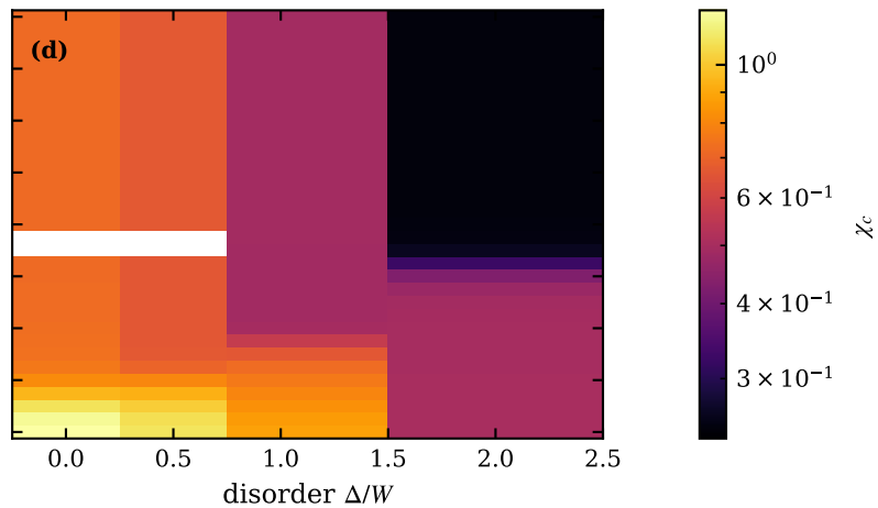
typ, n_c=0.4 , T/W=0.05 , \lambda=0
