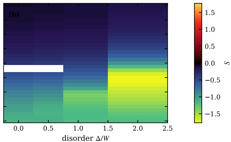
typ, n_c=0.24 , T/W=0.5 , \lambda=0
