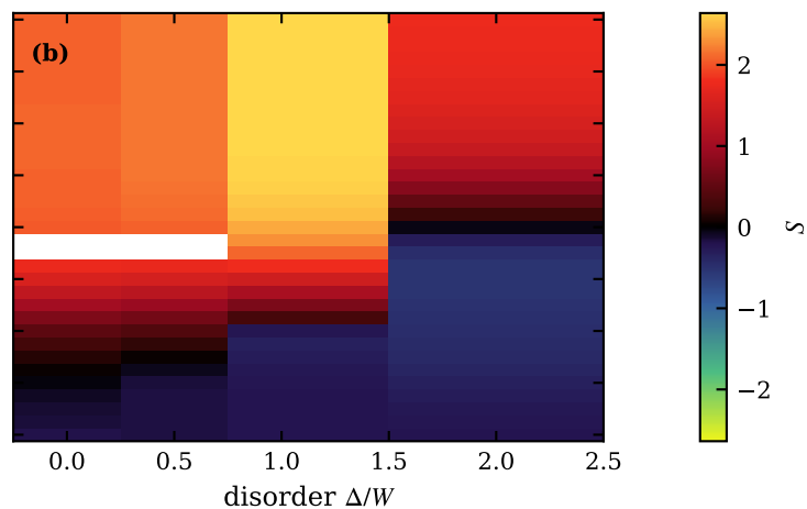
typ, n_c=0.45 , T/W=0.2 , \lambda=0
