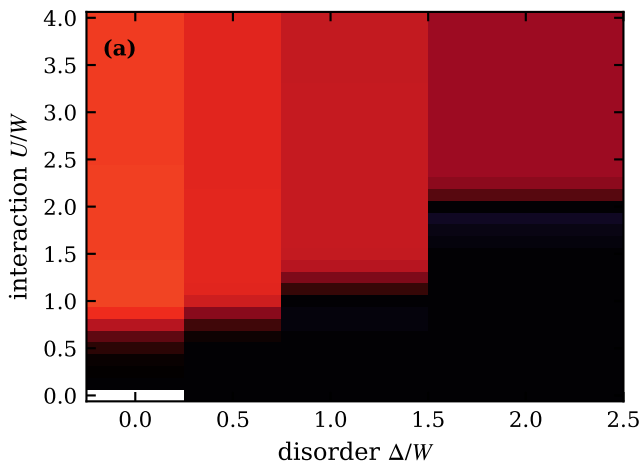
arith, n_c=0.49 , T/W=0.05 , \lambda=0
