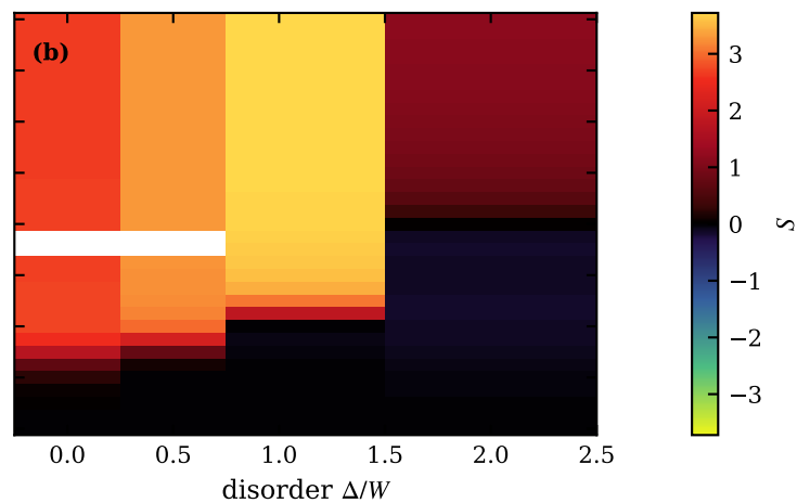
typ, n_c=0.49 , T/W=0.05 , \lambda=0
