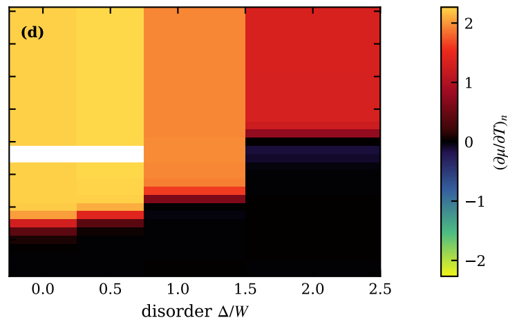
typ, n_c=0.49 , T/W=0.05 , \lambda=0
