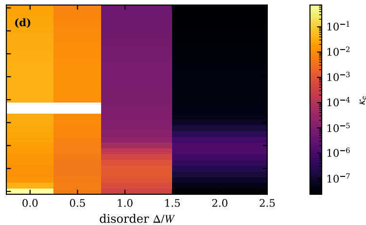
typ, n_c=0.49 , T/W=0.5 , \lambda=0
