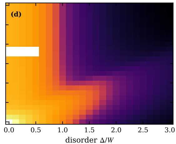
typ, n_c=0.3 , T/W=0.02
