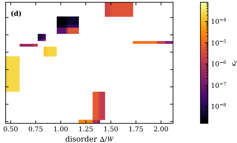
typ, n_c=0.5 , T/W=0.0075
