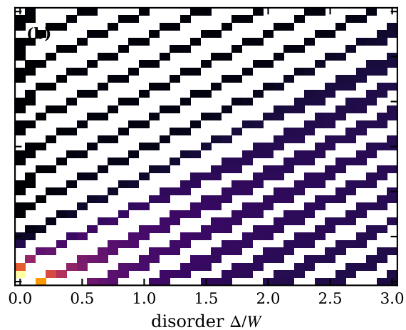
typ, n_c=0.4 , T/W=0.05 , \lambda=1
