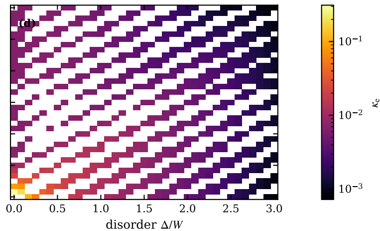
typ, n_c=0.4 , T/W=0.05 , \lambda=1.25
