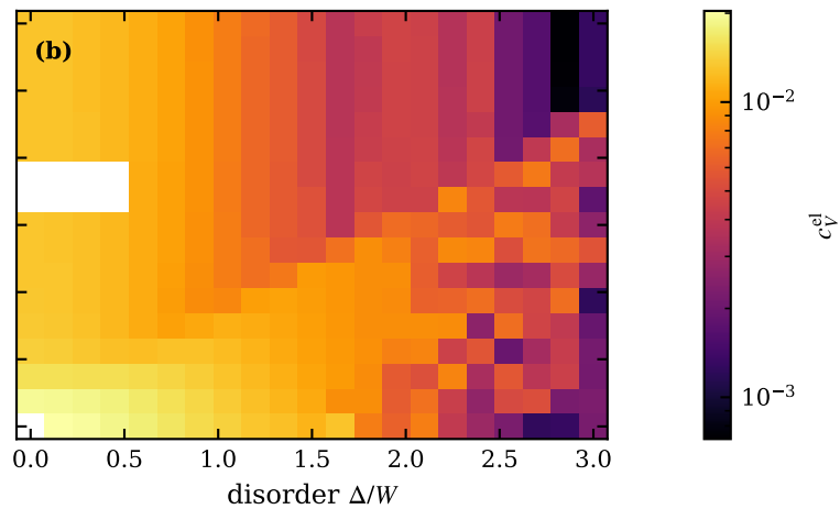
typ, n_c=0.4 , T/W=0.005
