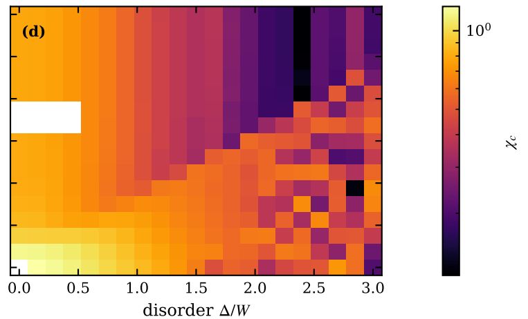
typ, n_c=0.4 , T/W=0.005
