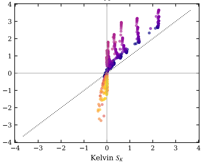
typ
