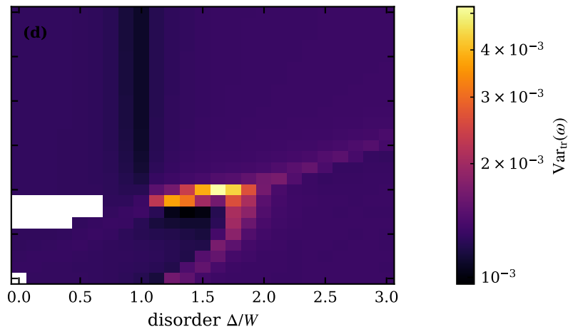
typ, n_c=0.25 , T/W=0.02
