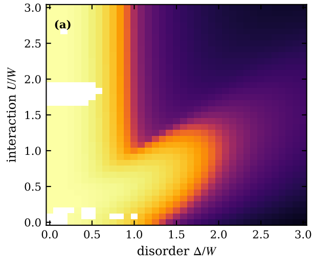
R_\sigma, n_c=0.4, T/W=0.5
