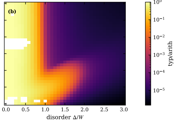
R_\kappa, n_c=0.4, T/W=0.5
