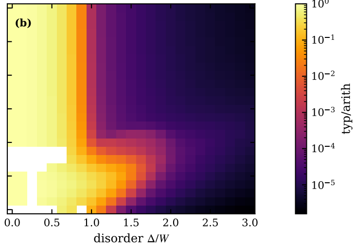
R_\kappa, n_c=0.2, T/W=0.05
