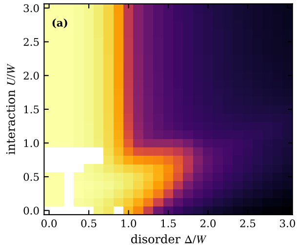
R_\sigma, n_c=0.2, T/W=0.05
