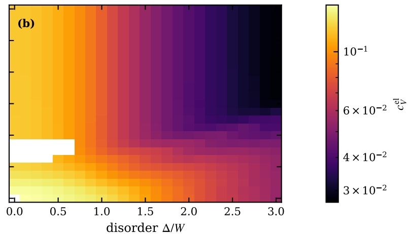
typ, n_c=0.2 , T/W=0.05
