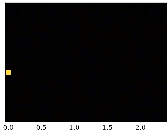
typ, n_c=0.5 , T/W=0.01
