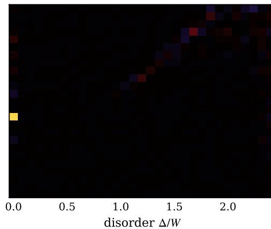
typ, n_c=0.5 , T/W=0.01
