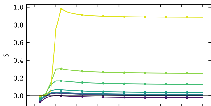
arith, T/W=0.05
