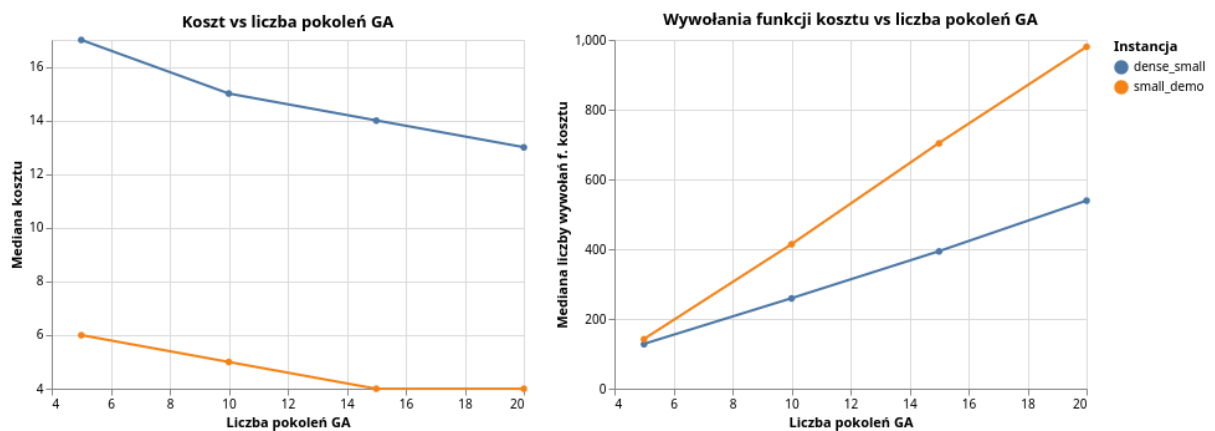
Rysunek 11: Wpływ liczby pokoleń na wynik algorytmu
