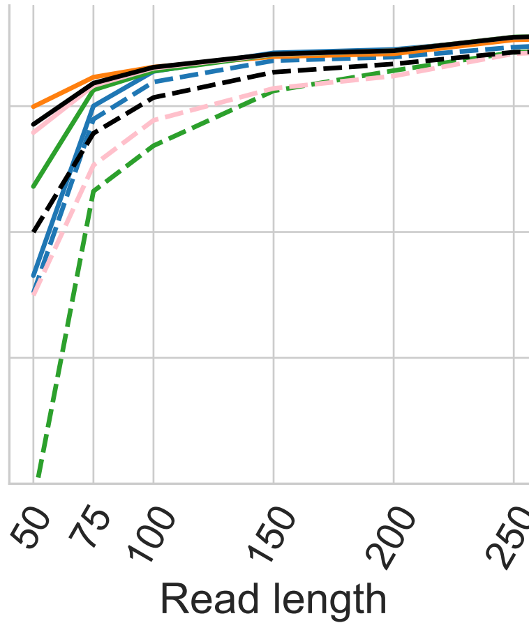
dataset = SIM4
