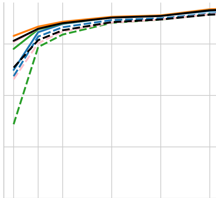
dataset = SIM2
