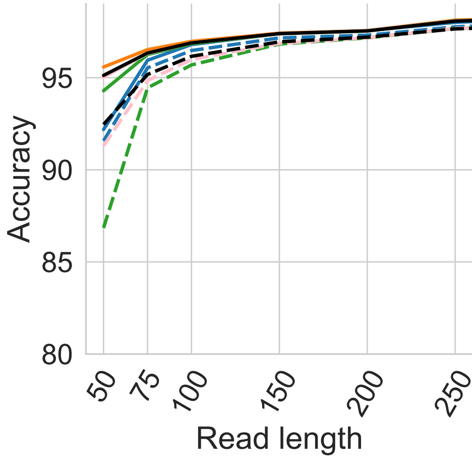
dataset = SIM3
