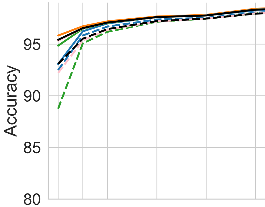
dataset = SIM1
