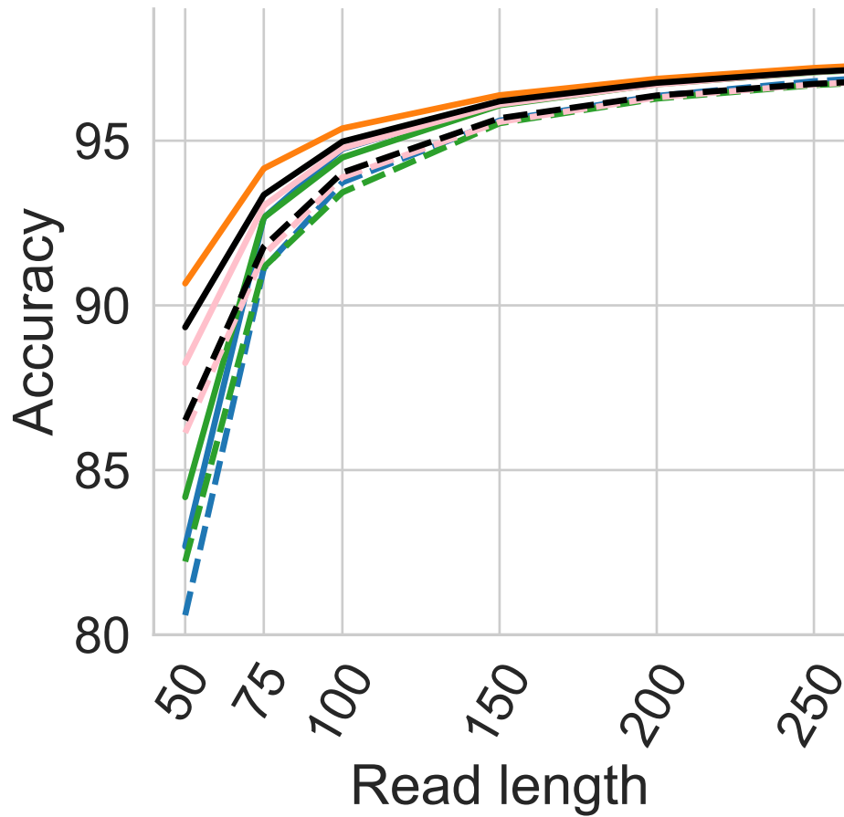
dataset = SIM3
