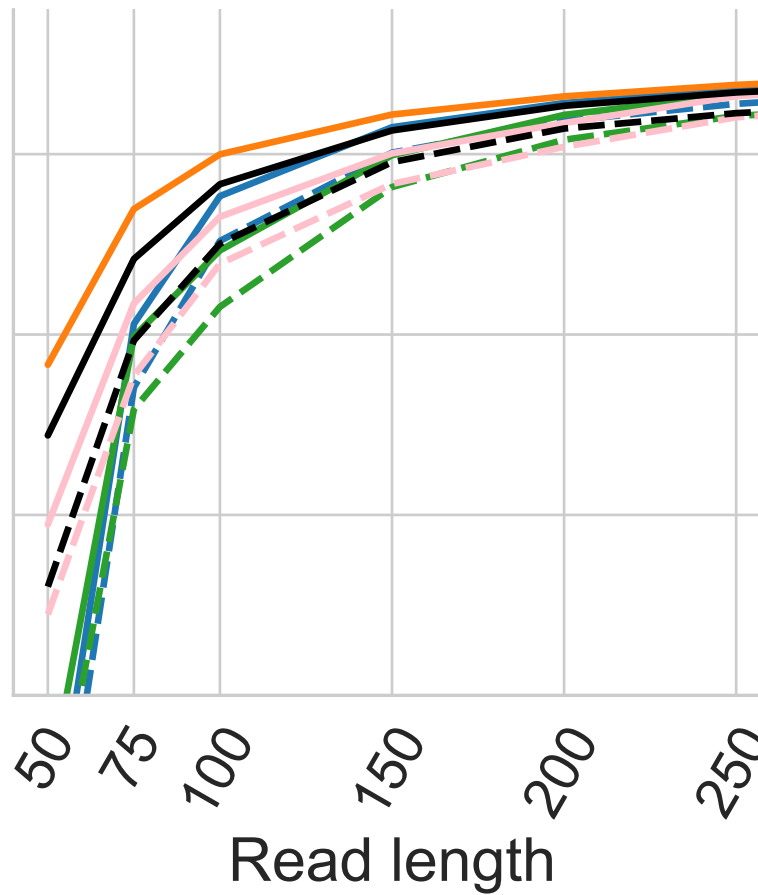
dataset = SIM4
