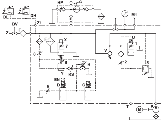
液压控制图
