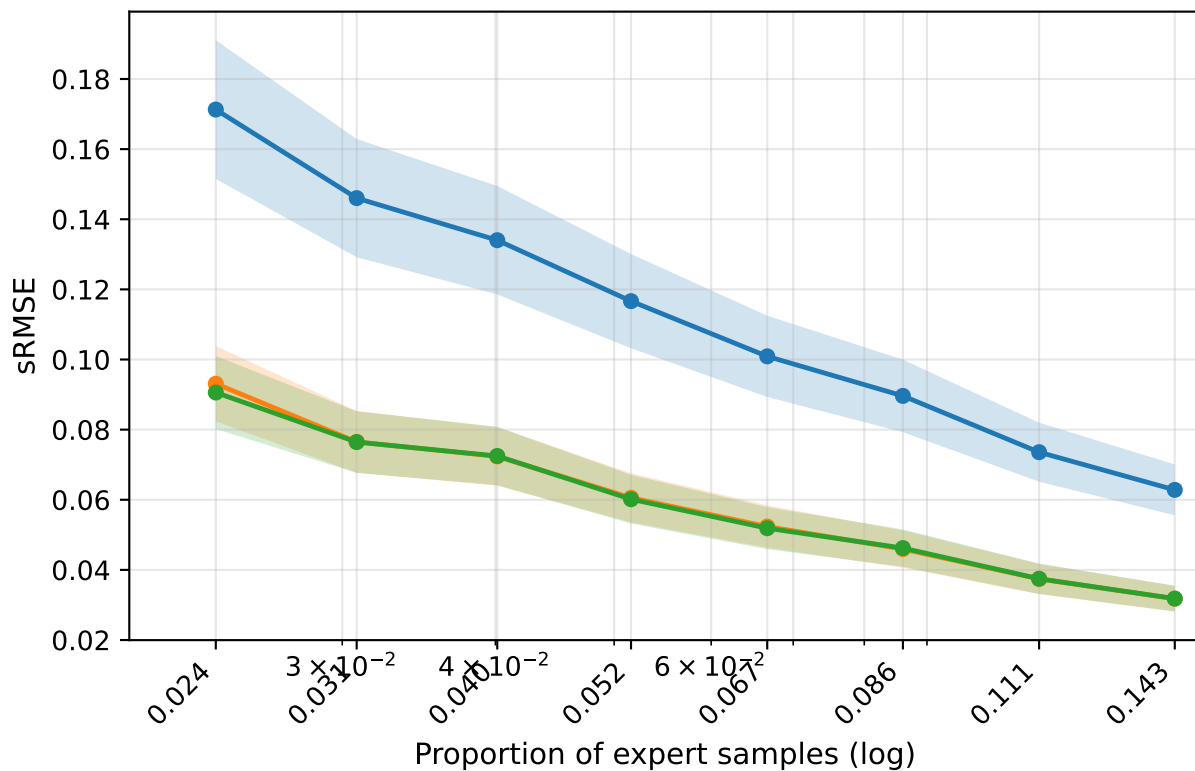
GPT-5.4
