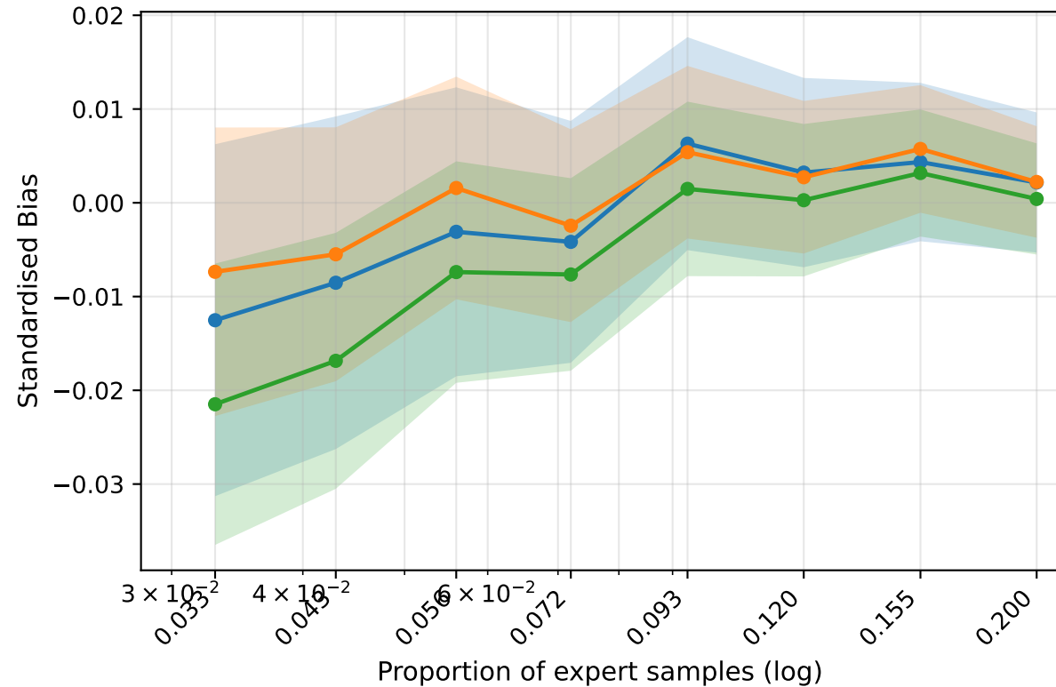
GPT-5.4
