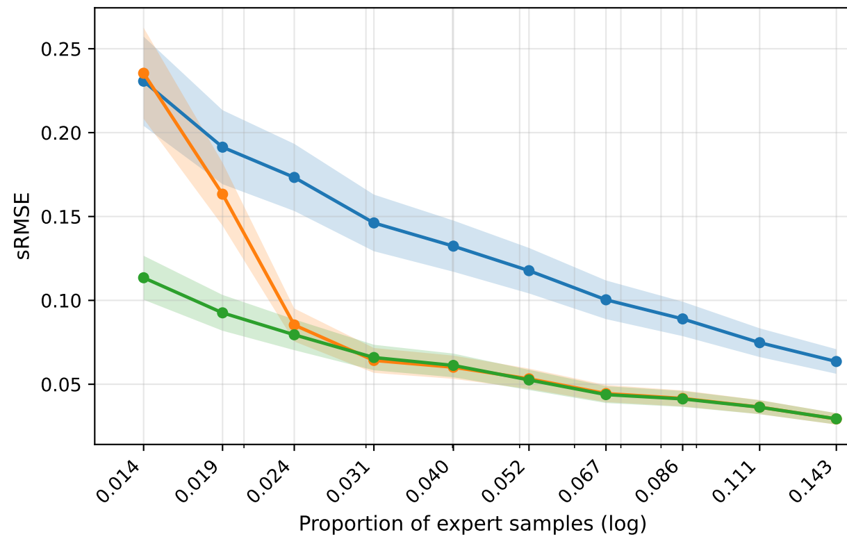
GPT-5.4
