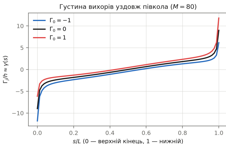
Рисунок 13: \Gamma_j/h \approx \gamma(s) (розд. 4.5): біля кінців густина різко зростає — клас «необмежений на обох кінцях» (розд. 4.5). При \Gamma_0 = 0 — антисиметрична.
