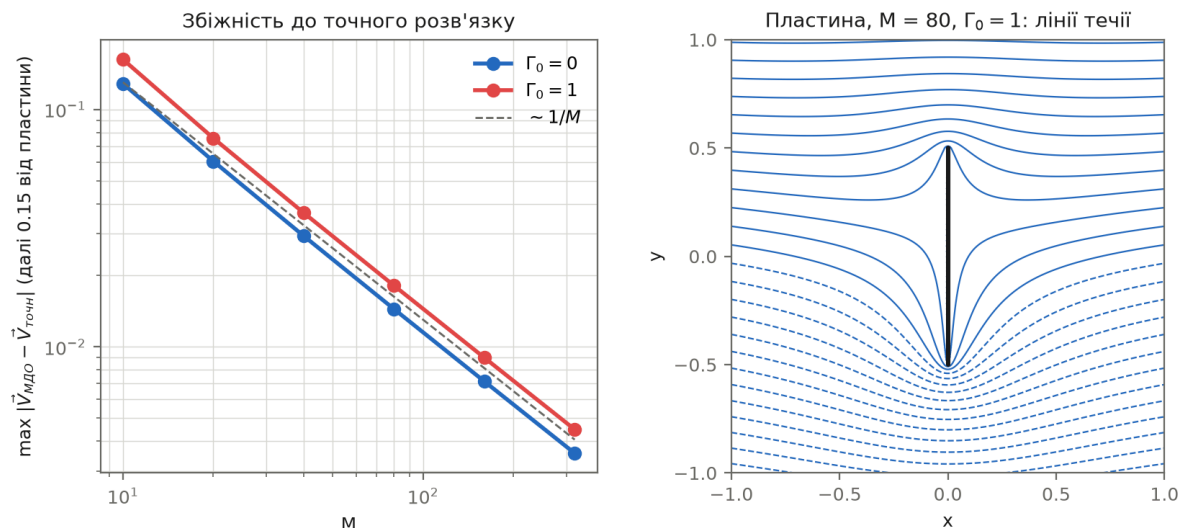
Рисунок 14: Ліворуч: похибка МДО відносно точного розв'язку спадає як 1/M . Праворуч: лінії течії навколо пластини, \Gamma_0 = 1 .
