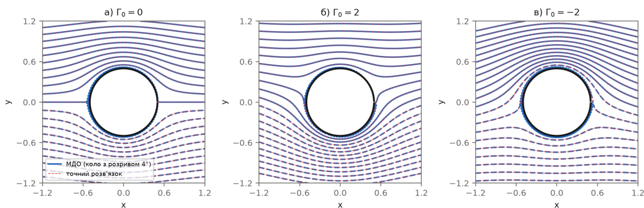
Рисунок 15: Коло з розривом 4^\circ , M = 80 : лінії течії МДО (суцільні) і точні (пунктир) збігаються. а/б/в — як на [Сл. 11, 14]: \Gamma_0 = 0, > 0, < 0 .
