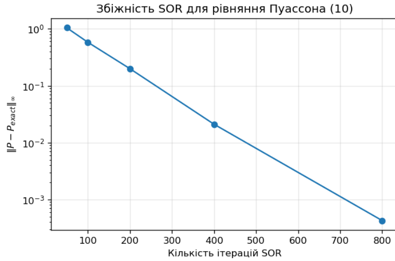
Рис. 5 – Збіжність SOR для рівняння Пуассона (тест з p_{\text{exact}} )
