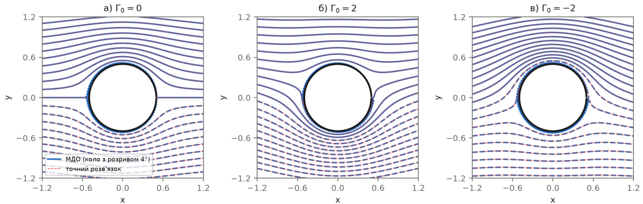
Рисунок 21: Коло з розривом 4^\circ , M = 80 : лінії течії МДО (суцільні) і точні (пунктир) збігаються. а/б/в — як на [Сл. 11, 14]: \Gamma_0 = 0, > 0, < 0 .
