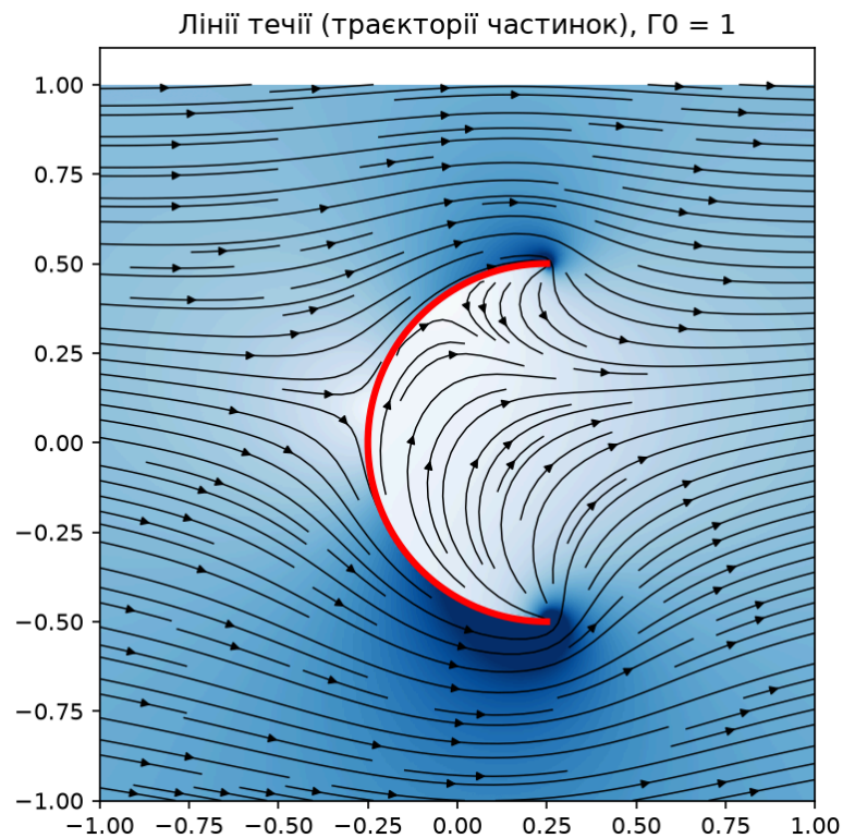
Рисунок 15: Лінії течії на тлі |\vec{V}| , \Gamma_0 = 1 .
