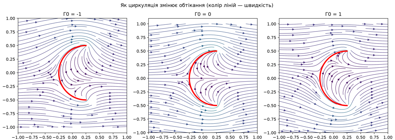
Рисунок 16: Ліворуч — закрученість за годинниковою стрілкою, у центрі — без неї (симетрично), праворуч — проти.
