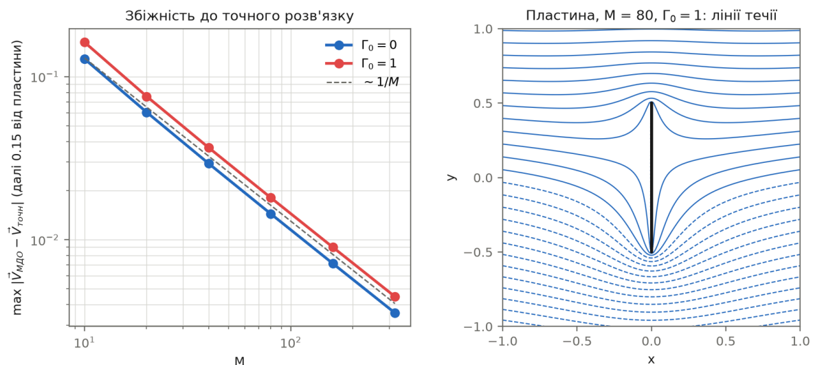
Рисунок 20: Ліворуч: похибка МДО відносно точного розв'язку спадає як 1/M . Праворуч: лінії течії навколо пластини, \Gamma_0 = 1 .
