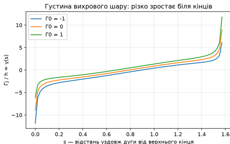
Рисунок 17: Густина вихрового шару для трьох \Gamma_0 .
