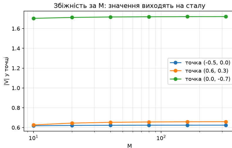
Рисунок 19: |\vec{V}| у трьох точках залежно від M .
