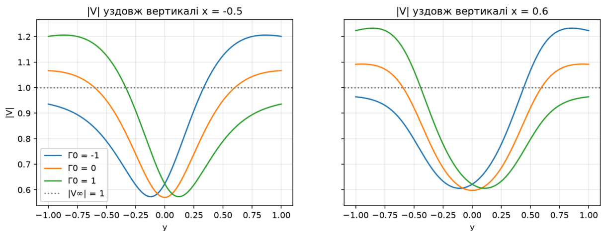
Рисунок 18: Модуль швидкості вздовж прямих x = -0.5 (перед перешкодою) і x = 0.6 (за нею).
