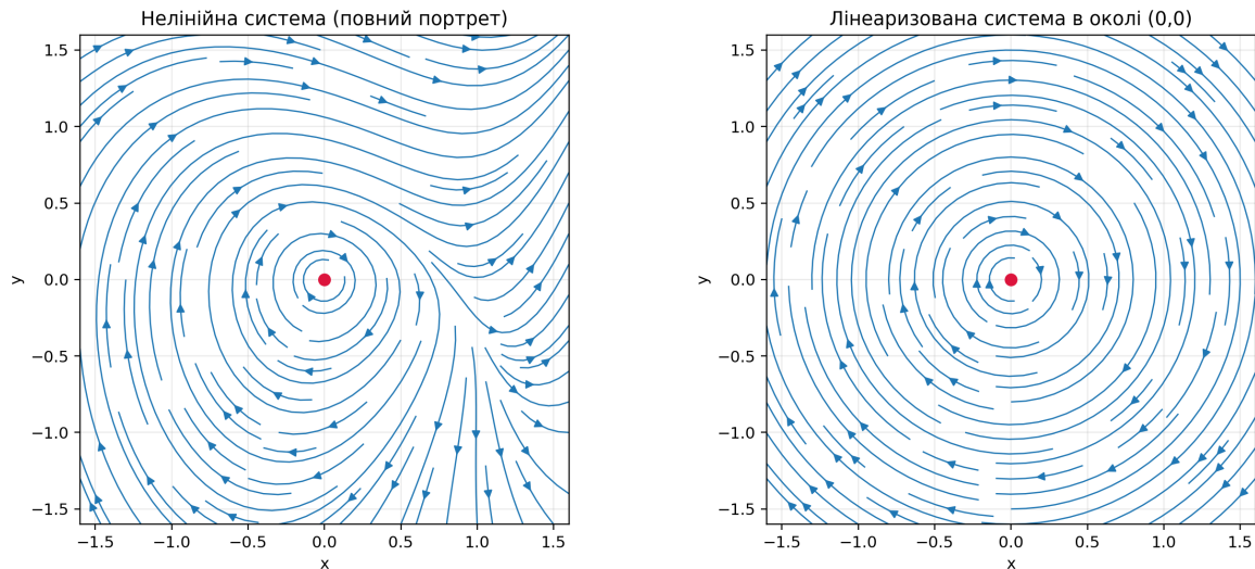
Рис. 1: Фазові портрети: нелінійна система (ліворуч) і лінеаризована система (праворуч).
