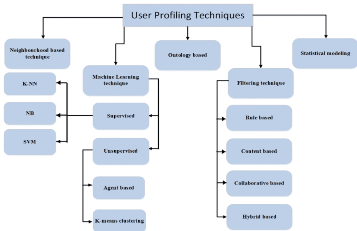
شکل ۱.۳: نمایش دهنده تکنیک‌های ساخت نمایه به تفکیک و همچنین روش‌های پیاده‌سازی هر تکنیک است [۳۰].
