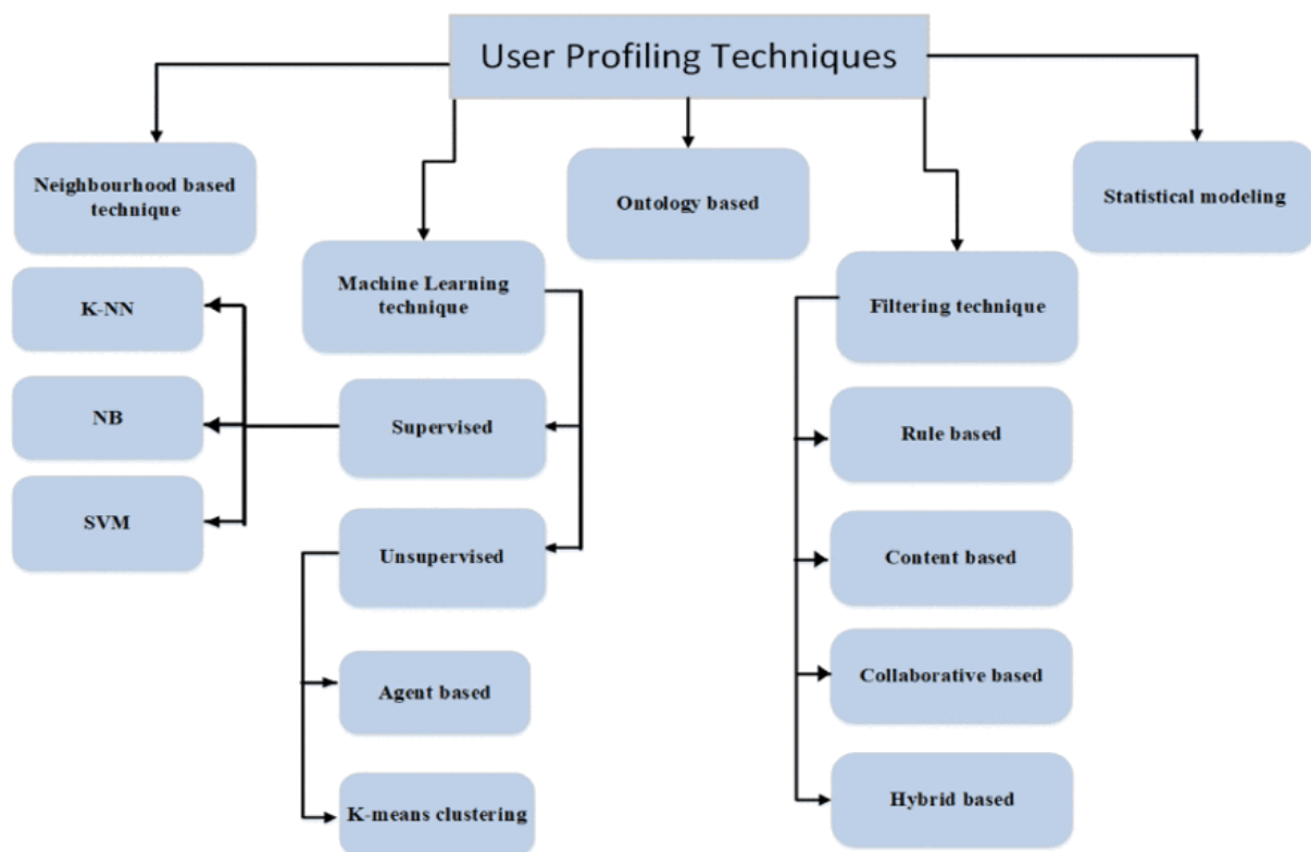
شکل ۱.۳: نمایش دهنده تکنیک‌های ساخت نمایه به تفکیک و همچنین روش‌های پیاده سازی هر تکنیک است [۲۸].
