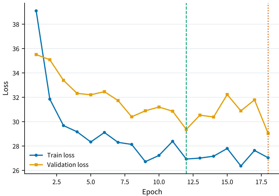
(a) 학습 및 검증 loss
