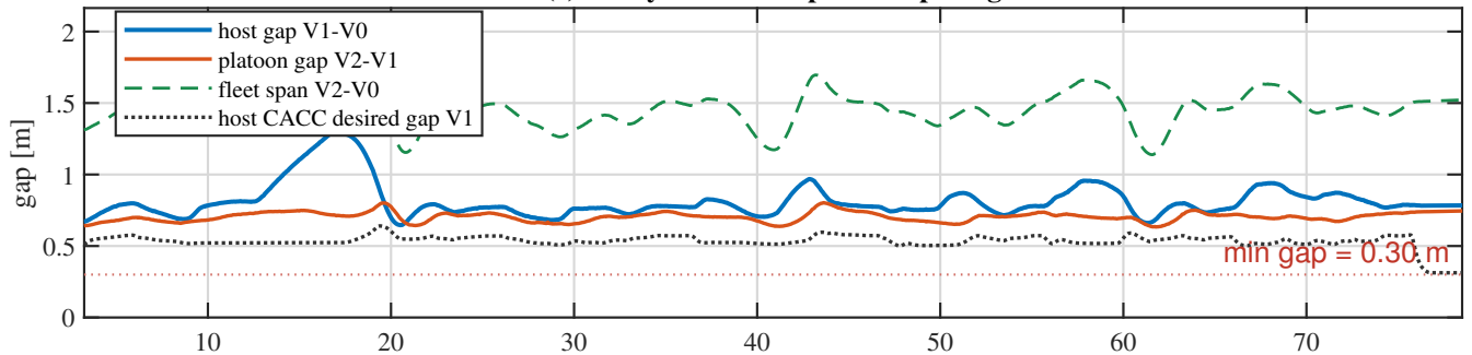
(d) V2V attack timeline
