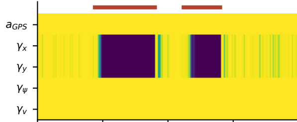
(d) GPS dropout
