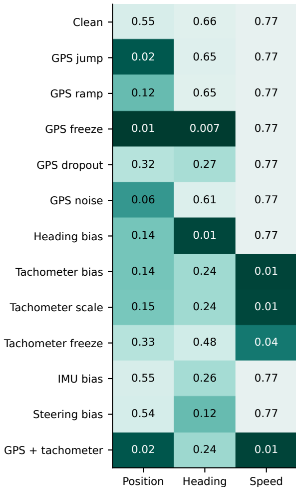
Hybrid / EKF
