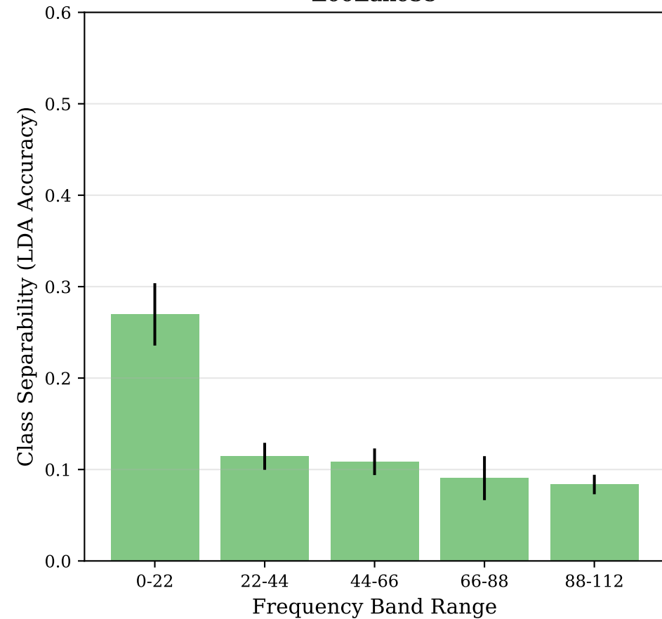
ZooLake35
