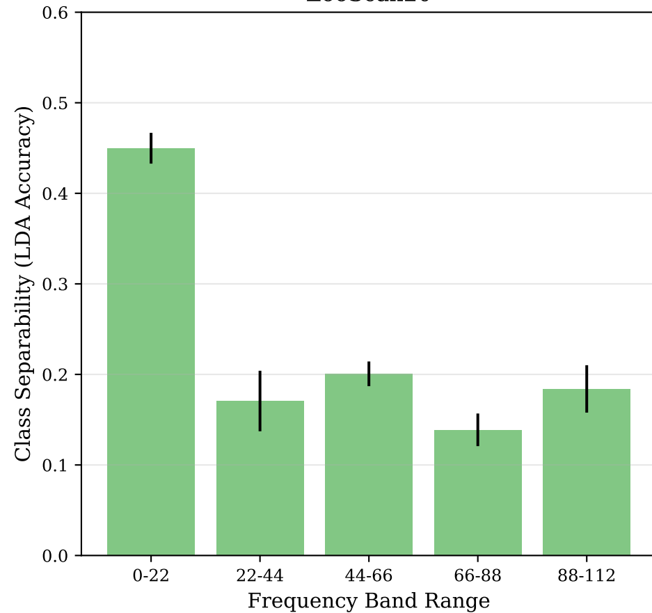
ZooScan20
