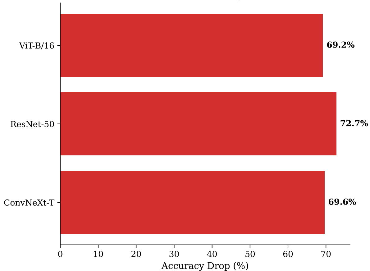
(b) Dataset shift magnitude
