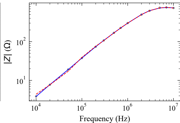
(d) TDK PC200
