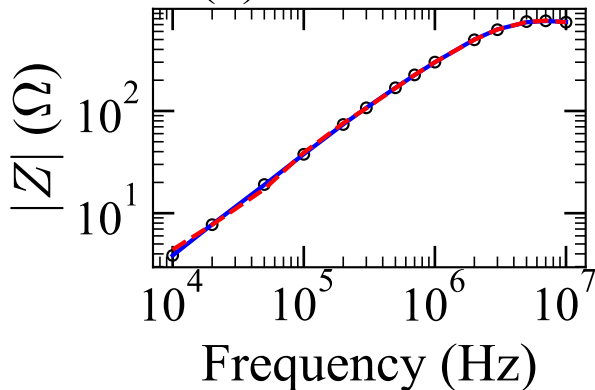
(d) TDK PC200
