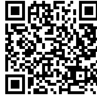
GitHub
