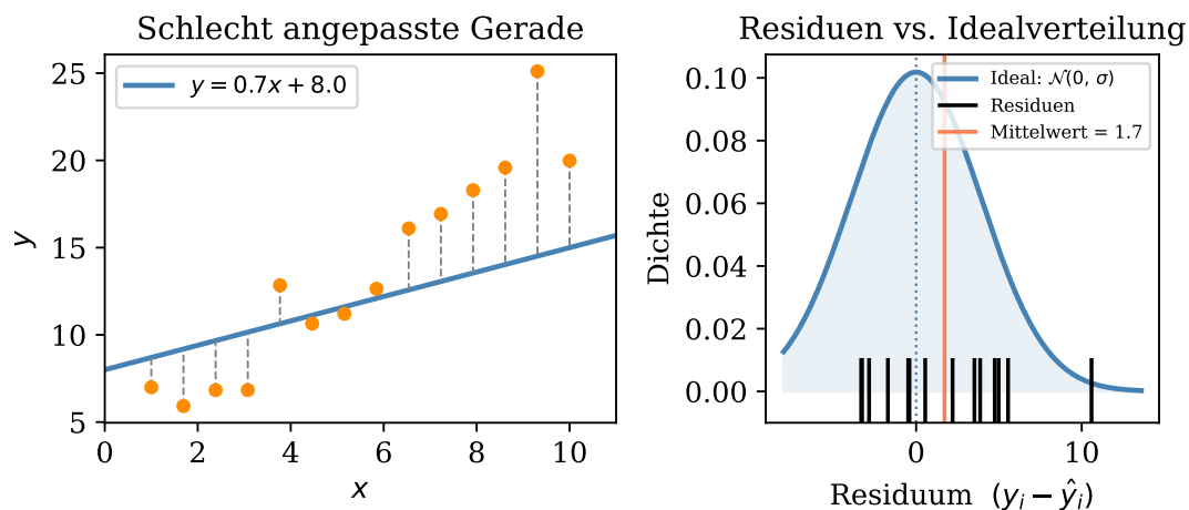
Abbildung 1: Links: Schlecht gewählte Gerade ( y = 0,7x + 8 ), gestrichelte Linien zeigen die Residuen. Rechts: Die Residuen (schwarze Striche) unter der idealen \mathcal{N}(0, \sigma) -Verteilung – ihr Mittelwert liegt deutlich von Null entfernt, die Likelihood ist niedrig .
