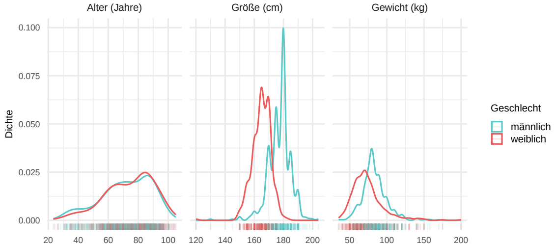
Abbildung: Kerndichteschätzungen mit Gaußkern für Alter, Größe und Gewicht.
