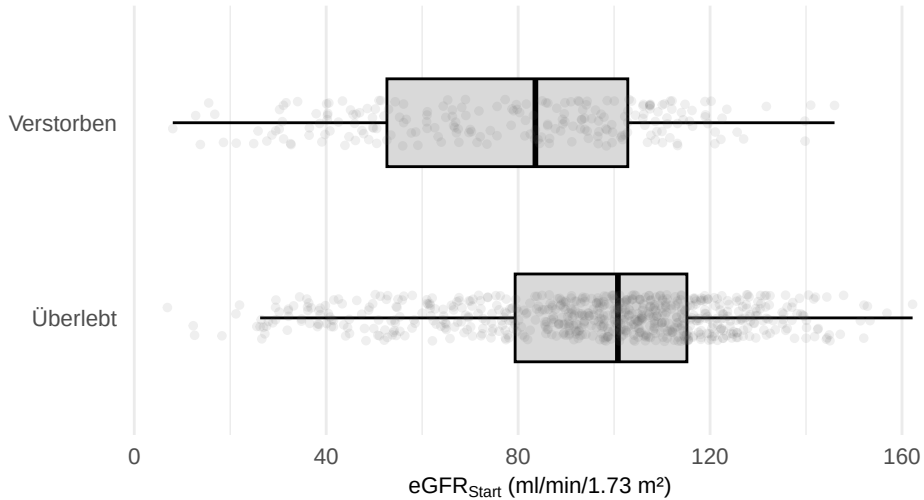
Abbildung: Verteilung von eGFR_{Start} nach Mortalitätsstatus.
