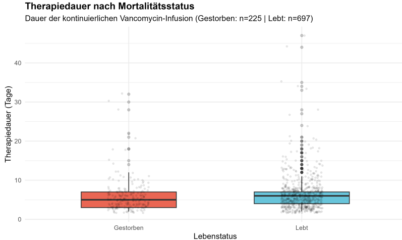
Abbildung: Dauer der Vancomycin-Therapie nach Mortalitätsstatus.
