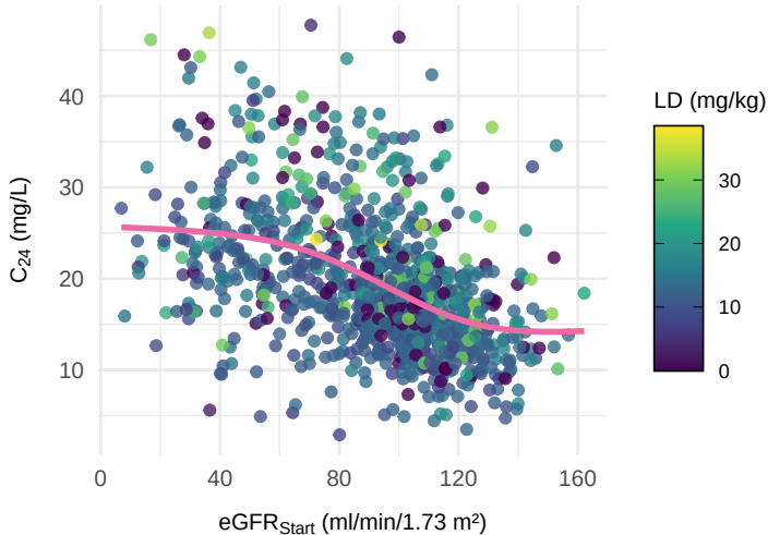
Abbildung: Zusammenhang zwischen Vancomycin-Serum-Spiegel nach 24h ( C_{24} ) und der geschätzten glomerulären Filtrationsrate zu Beginn der Therapie( eGFR_{Start} ) (GAM-Trend).
