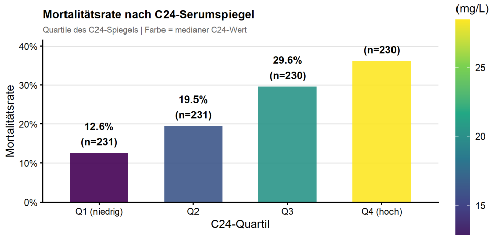
Abbildung: Mortalitätsrate nach Quartilen des Vancomycin-Serumspiegels (C24).
