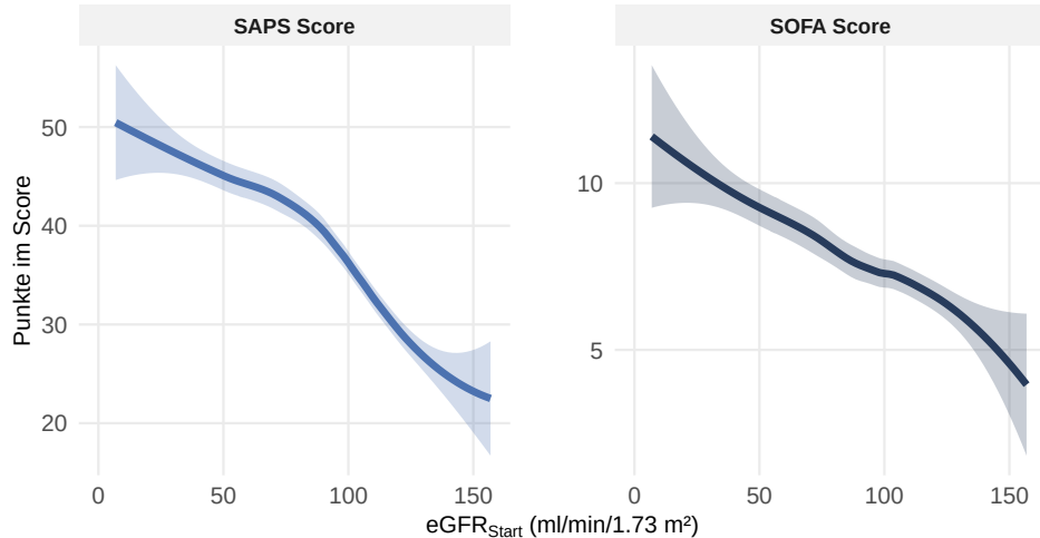
Abbildung: Korrelation von eGFR_{Start} zum SAPS- und SOFA-Score mit LOESS-Trendlinie und 95 % Konfidenzintervall.
