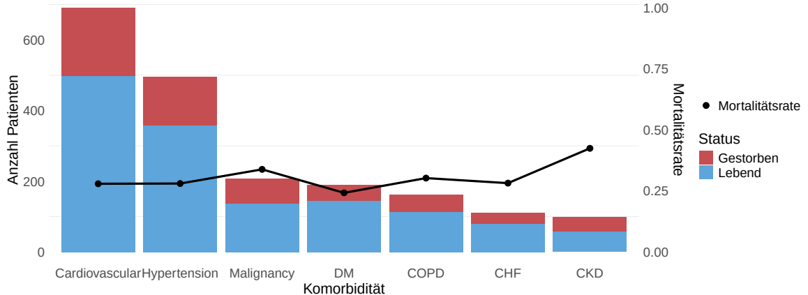
Abbildung: Barplot Anzahl von Patienten und Mortalitätsrate abhängig von Komorbiditäten.
