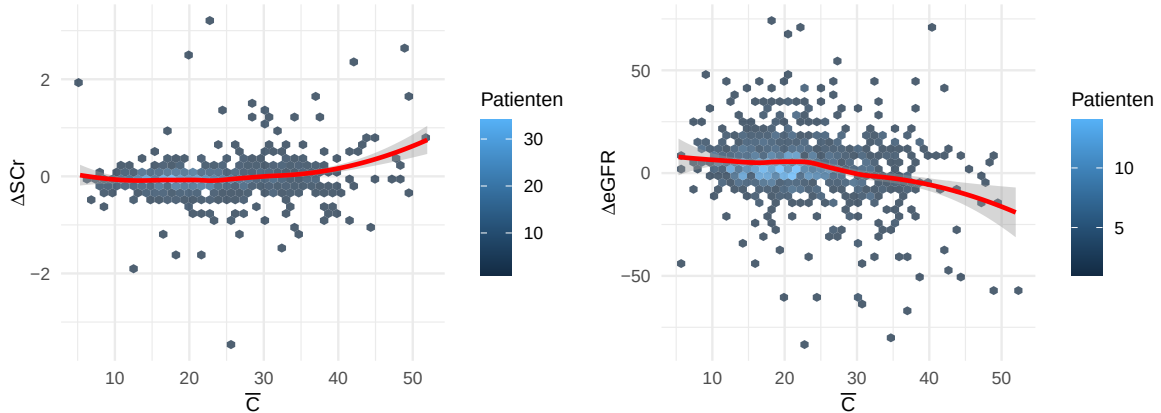
Abbildung: Hexbin-Plots von \Delta\text{SCr} und \Delta\text{eGFR} gegen die mittlere Vancomycin-Konzentration ( \bar{C} ) mit LOESS-Trendlinie.
