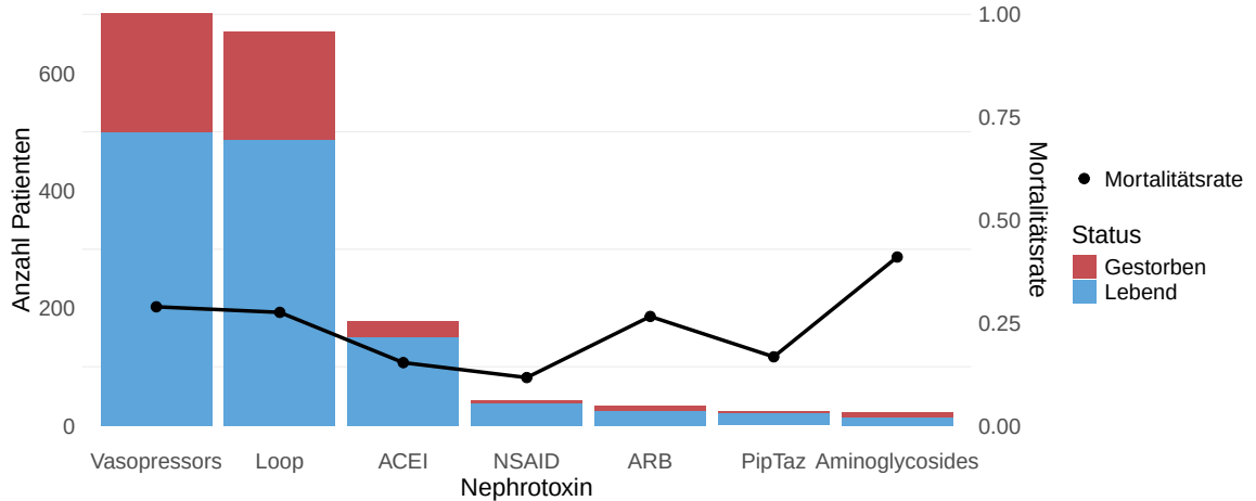
Abbildung: Barplot Anzahl von Patienten und Mortalitätsrate abhängig von Nephrotoxinen.
