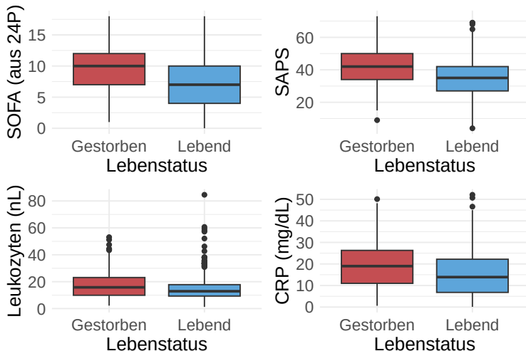
Abbildung: Boxplots der Schweregradvariablen zu Therapiebeginn (erste 24h), gruppiert nach Mortalitätsstatus (lebt vs. gestorben).
