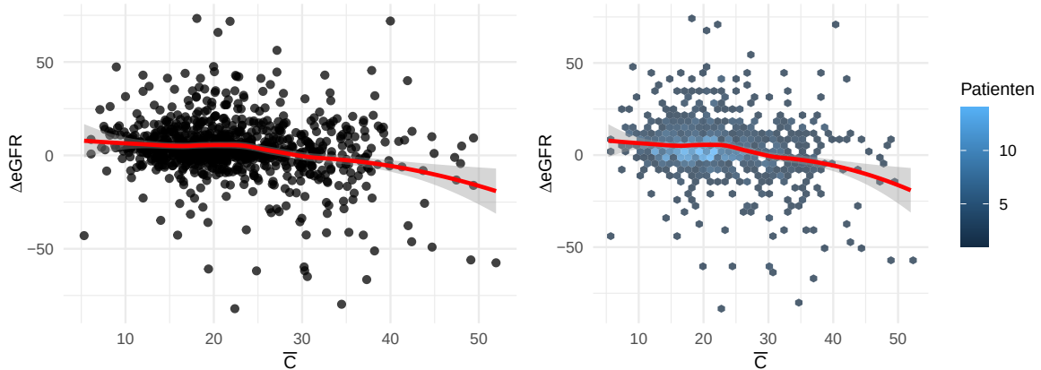
Abbildung: Vergleich der Darstellung desselben Datensatzes als Scatterplot und Hexbin-Plot.
