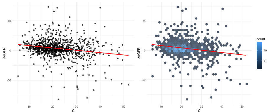
Abbildung: Vergleich der Darstellung desselben Datensatzes als Scatterplot und Hexbin-Plot.
