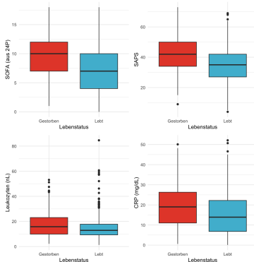
Abbildung: Boxplots der Schweregradvariablen zu Therapiebeginn (erste 24h), gruppiert nach Mortalitätsstatus (lebt vs. gestorben).
