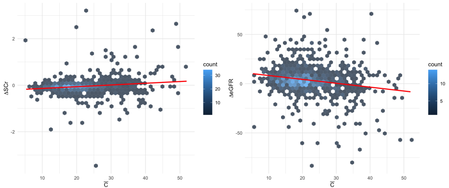
Abbildung: Hexbin-Plots von SCr und eGFR in Abhängigkeit von der mittleren C-Konzentration ( \bar{C} ).
