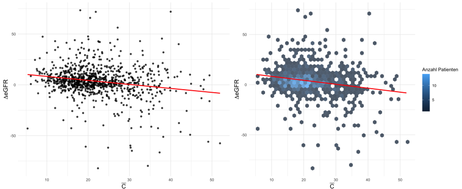
Abbildung: Vergleich der Darstellung desselben Datensatzes als Scatterplot und Hexbin-Plot.
