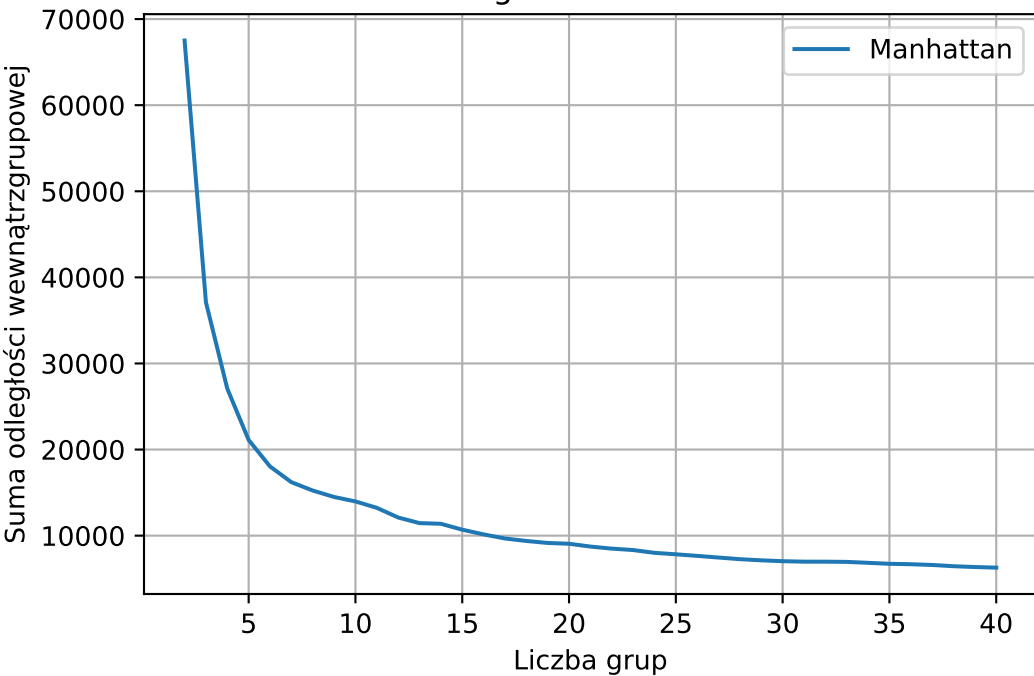
Odległość manhattan
