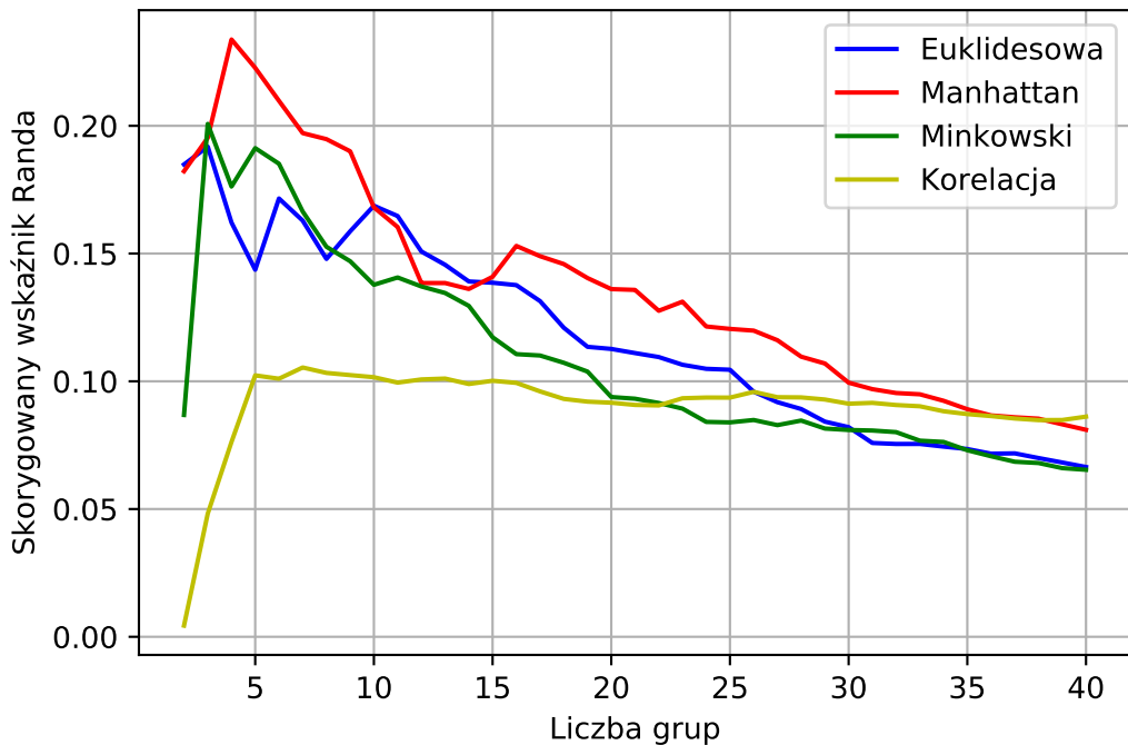
Skorygowany wskaźnik Randa
