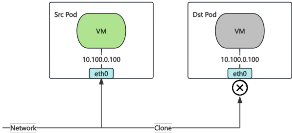
1. KubeVirt VM
